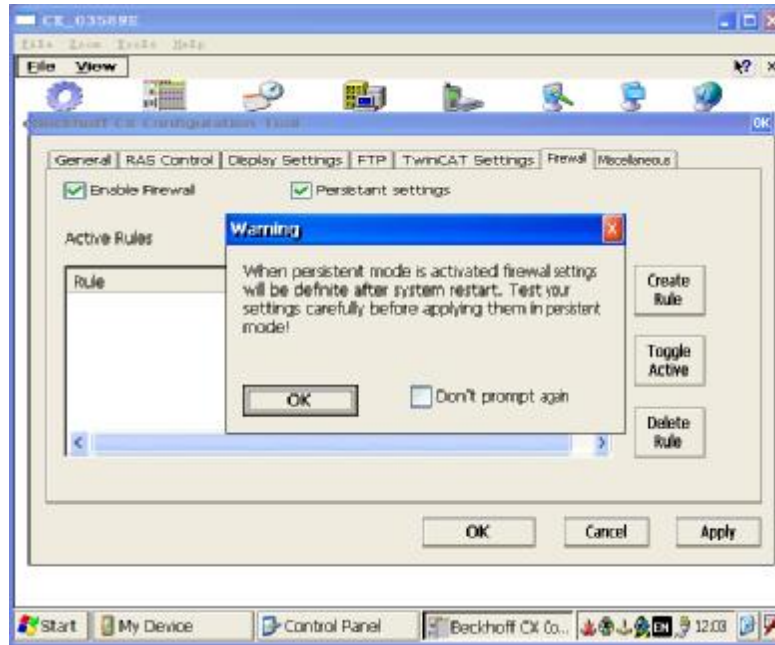
图A22 激活防火墙，并且设置为永久有效
