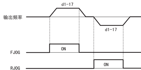
图 5.43 点动运行曲线
