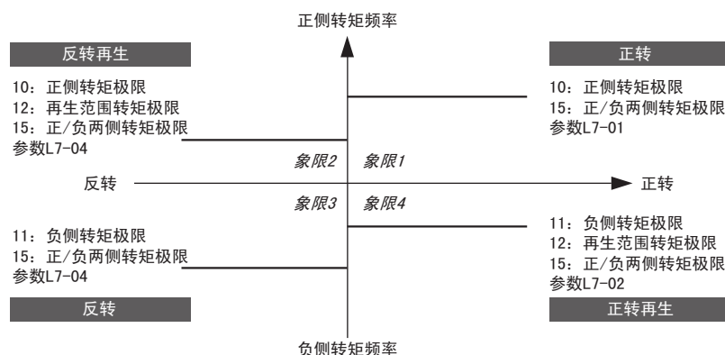
图 5.66 模拟量输入的转矩极限
