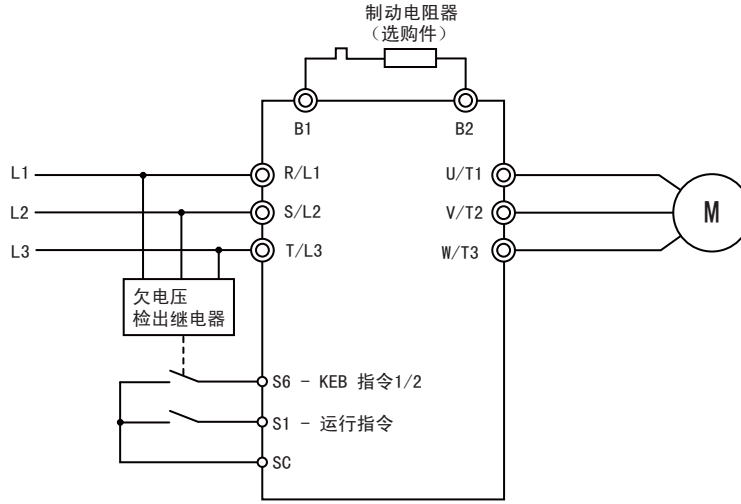
图 5.73 KEB 功能的接线示例
