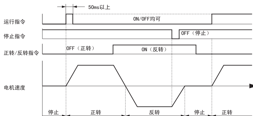
图 5.40 3 线制顺控的时序图
