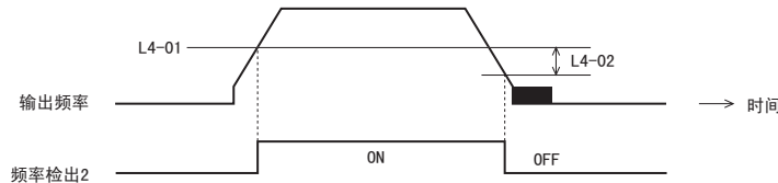
图 4.11 频率检出 2
