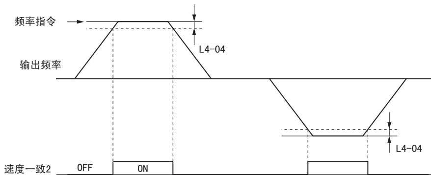
图 5.54 速度一致 2 的时序图
