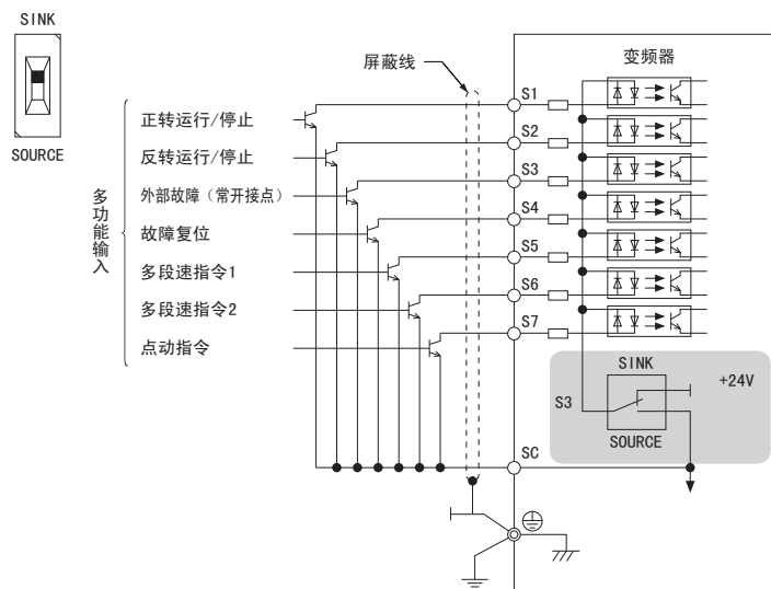
图 3.28 与 0V 公共点 / 共发射极模式下的 NPN 晶体管的连接示例
