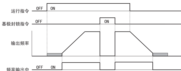
图 5.59 频率输出中的时序图
