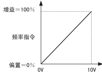
图 5.62 模拟量输入端子 A1 的特点（出厂设定）
