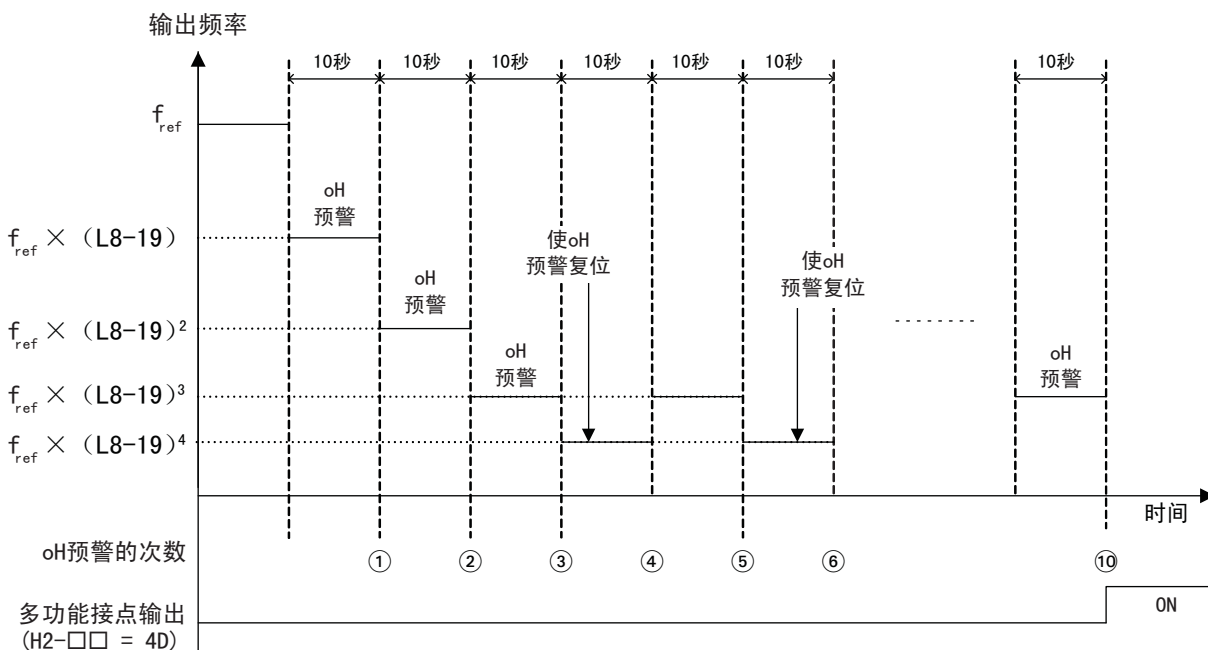
图 5.81 散热片过热预警输出时输出频率的递减动作
