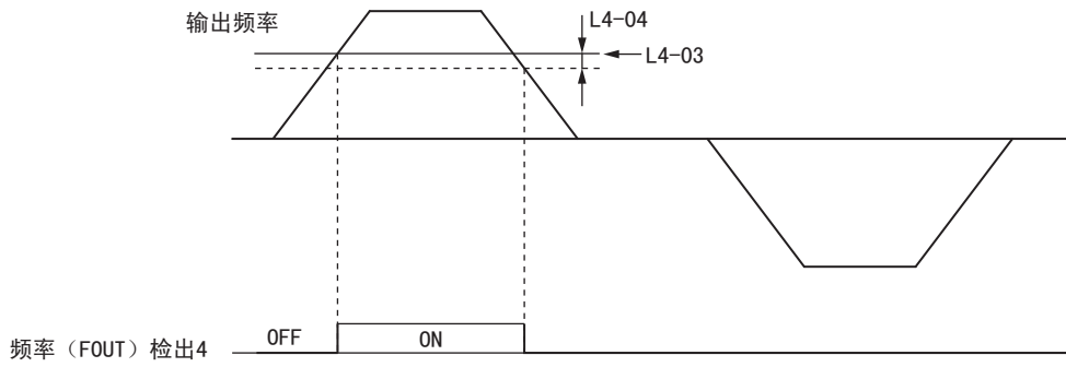
图 5.57 频率 (FOUT) 检出 4 的示例 (L4-03 为正时)
