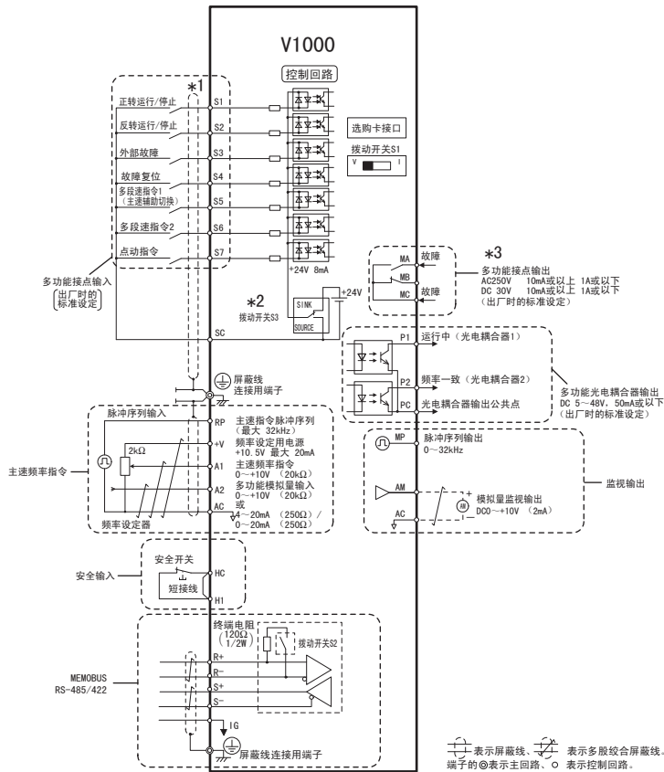
图 3.20 控制回路连接图
