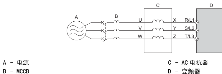
图 8.3 AC 电抗器的连接示例
