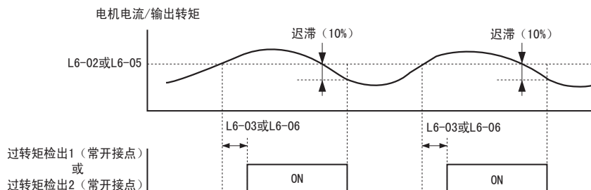
图 5.79 过转矩检出的时序图
