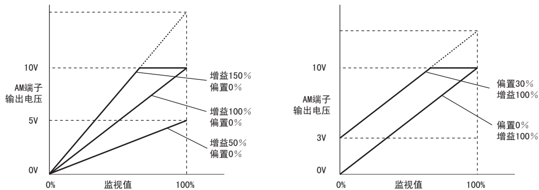
图 5.67 模拟量输出的增益 / 偏置设定
