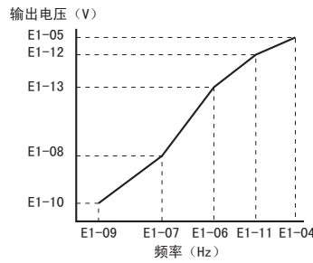
图 5.36 V/f 曲线图
