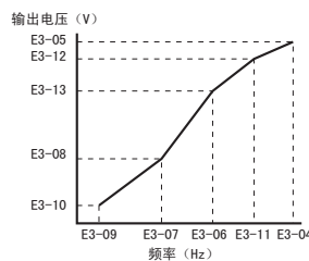
图 5.37 电机 2 的 V/f 曲线图
