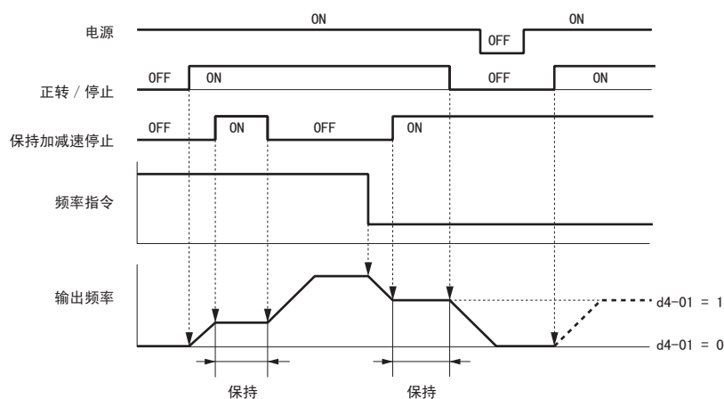
图 5.30 频率指令保持和保持加减速停止功能
