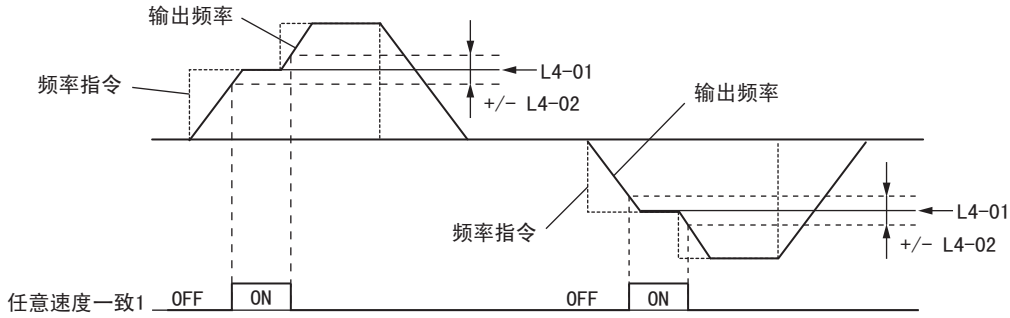
图 5.51 任意速度一致 1 的时序图
