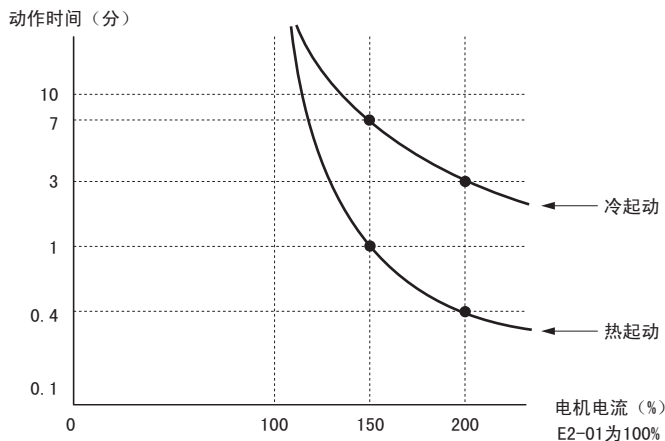
图 5.69 电机保护动作时间
