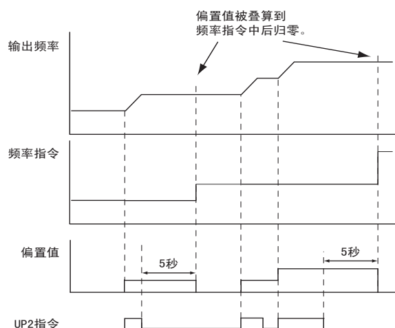
图 5.31 UP2/DOWN2 指令和从 LED 操作器输入的频率指令的组合 (d4-01 = 1)
