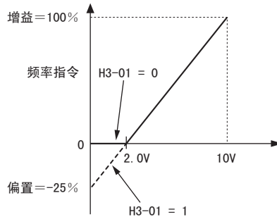
图 5.64 设定了负值偏置时的频率指令
