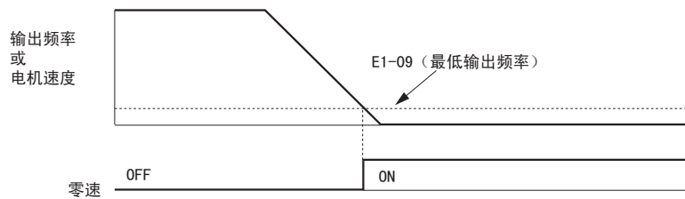
图 5.49 零速的时序图
