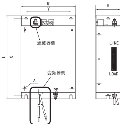
图 D.7 EMC 噪音滤波器的外形尺寸
