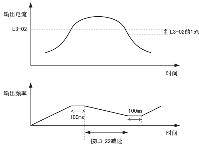
图 5.75 PM 用无 PG 矢量控制时的加速中防止失速功能
