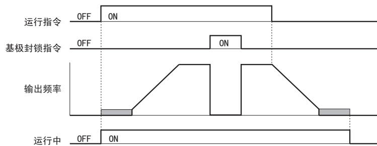
图 5.48 运行中的时序图
