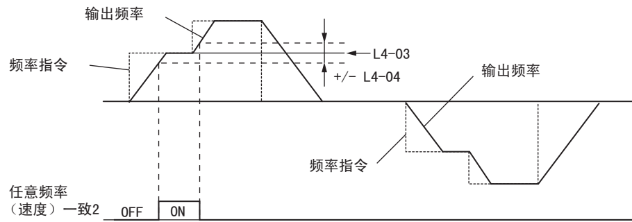
图 5.55 任意频率（速度）一致 2 的示例（L4-03 为正时）
