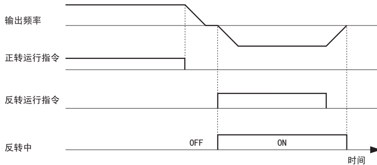
图 5.58 反转中输出时序图
