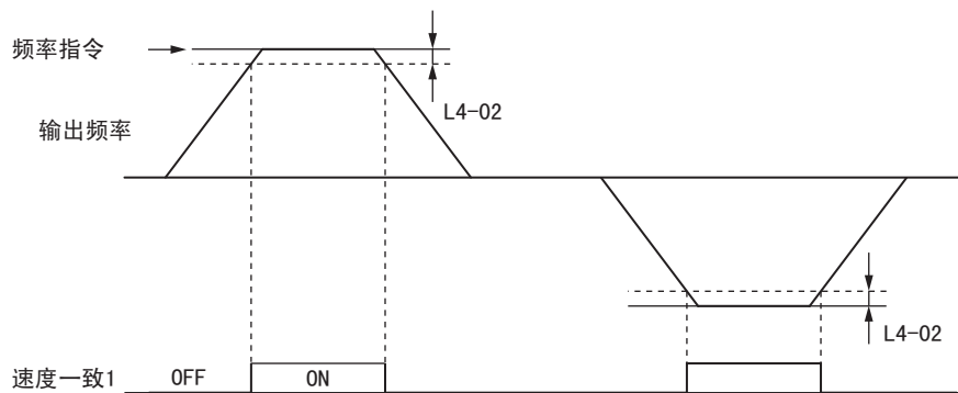
图 5.50 速度一致 1 的时序图
