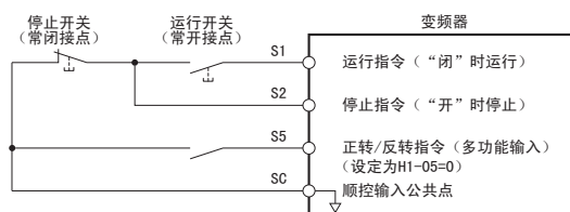
图 3.2 3 线制顺控
