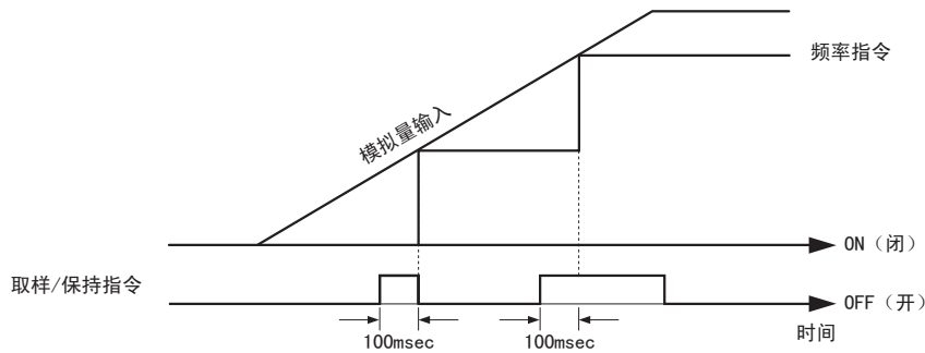
图 5.46 模拟量频率指令的取样 / 保持
