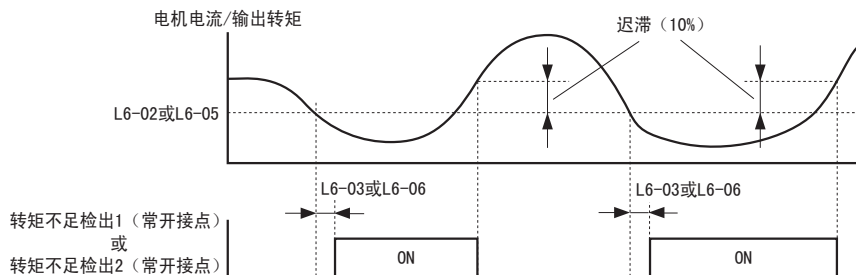
图 5.80 转矩不足检出的时序图
