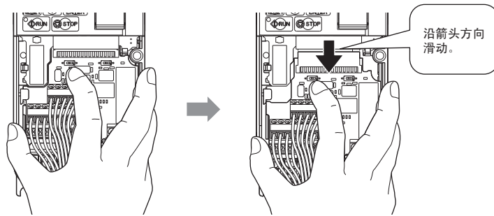
图 7.8 端子排的拆卸
