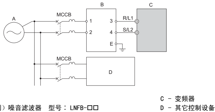
图 8.5 输入侧（一次侧）噪音滤波器的连接示例（单相 200V）
