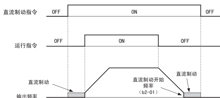
图 5.47 直流制动的时序图
