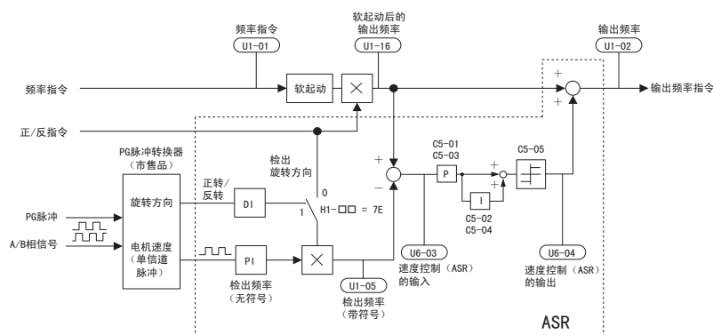
图 5.23 简易带 PG 速度控制框图
