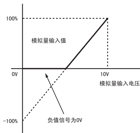
图 5.60 有 0 极限的模拟量输入（偏置设定 -100%）
