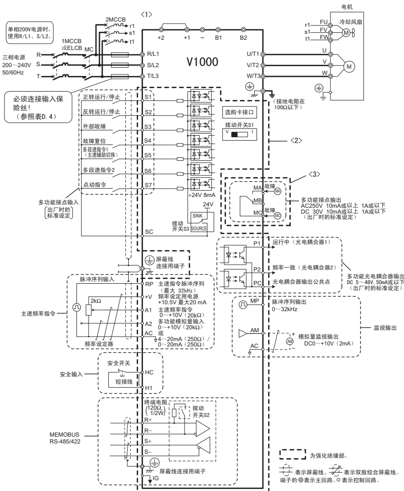
图 D.2 符合低电压指令的相互接线图 (200V 级示例)
