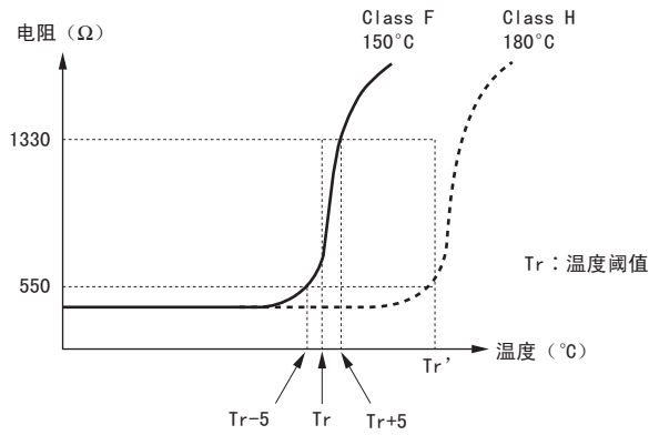
图 5.71 PTC 热敏电阻的温度 - 阻值特性
