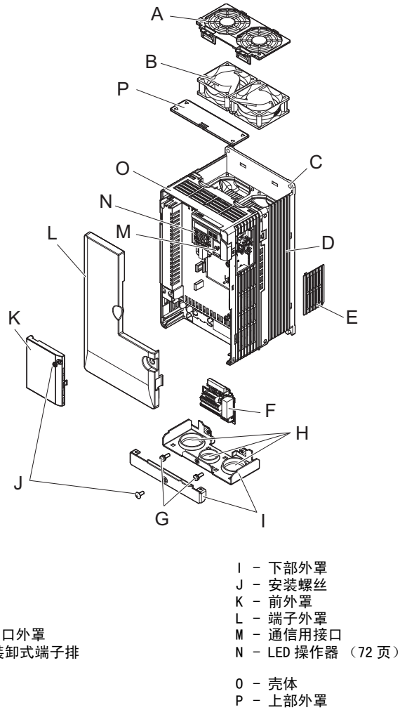
图 1.4 封闭壁挂型变频器各部分的名称 CIMR-V□4A0018F
