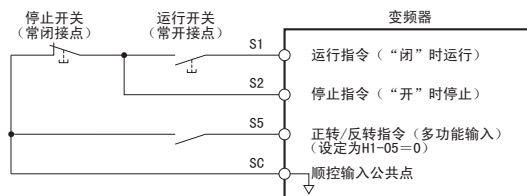
图 5.39 3 线制顺控的接线示例
