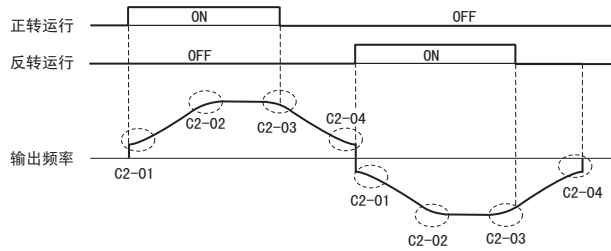
图 5.21 正转 / 反转切换时的 S 字特性
