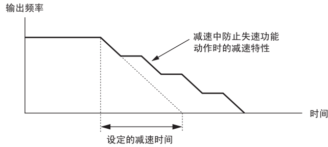
图 5.77 减速中防止失速的动作示例
