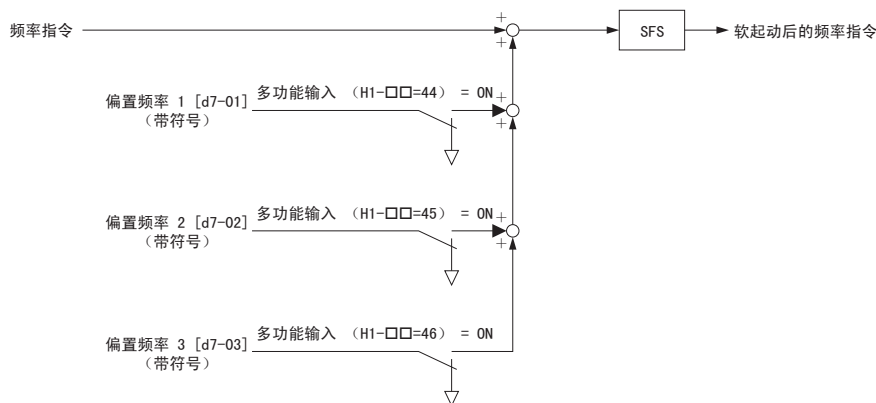
图 5.35 偏置频率框图
