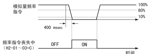
图 5.78 频率指令丧失时的功能
