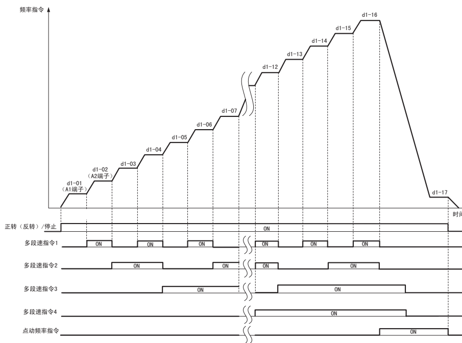
图 5.27 多段速指令 / 点动频率选择的时序图
