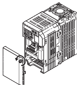
图 3.10 前外罩的拆卸方法（柜内安装型：IP20）
