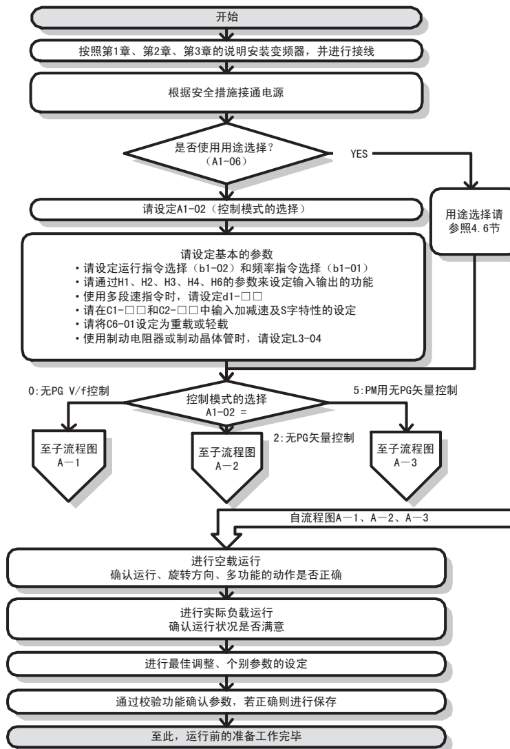
图 4.7 基本设定与电机调整
