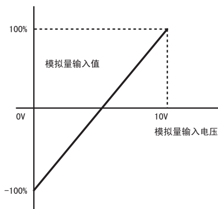
图 5.61 无 0 极限的模拟量输入（偏置设定 -100%）
