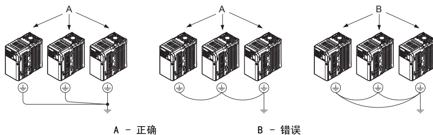
图 3.19 多台变频器的接线
