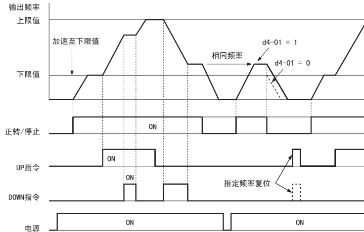
图 5.42 UP/DOWN 指令的时序图
