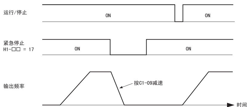
图 5.44 紧急停止的时序图
