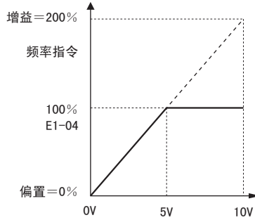
图 5.63 调整了模拟量输入的增益设定时的频率指令
