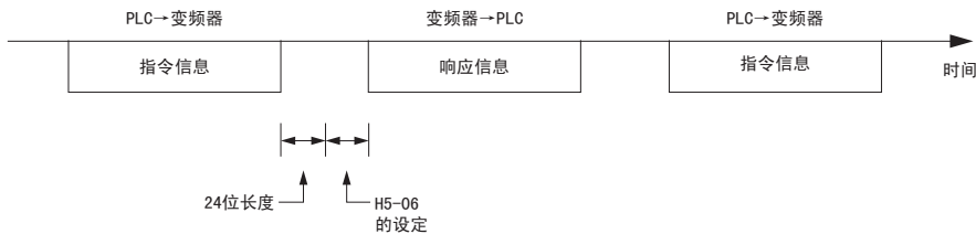
图 C.8 响应等待时间
