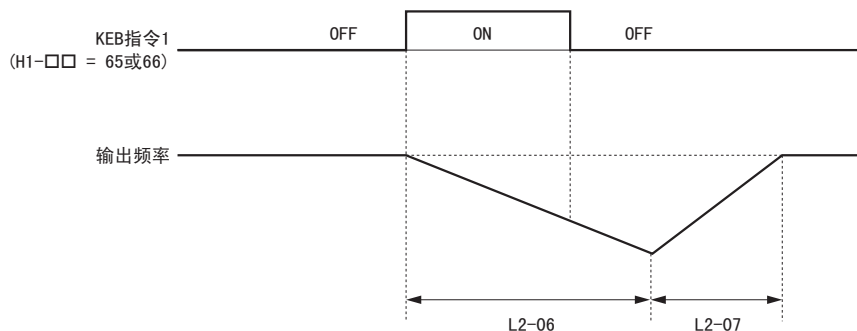
图 5.72 指令 1 的时序图
