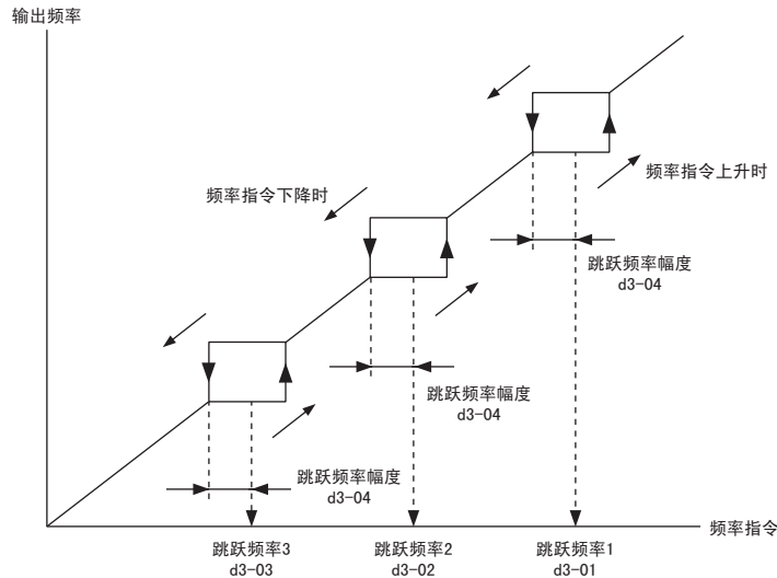
图 5.29 跳跃频率
