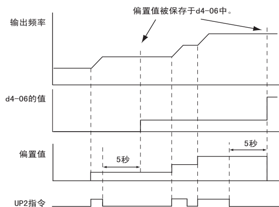
图 5.32 UP2/DOWN2 指令和从操作器以外输入的频率指令的组合 (d4-01 = 1)
