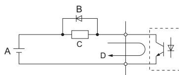
A - 外部电源 48V 或以下 B - 旁路二极管 C - 线圈 D - 50mA 或以下
