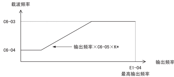
图 5.25 与输出频率相应的载波频率的变化
