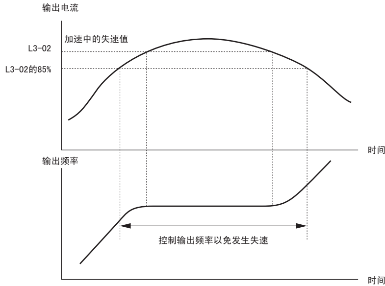
图 5.74 使用感应电机时的加速中防止失速功能的时序图
