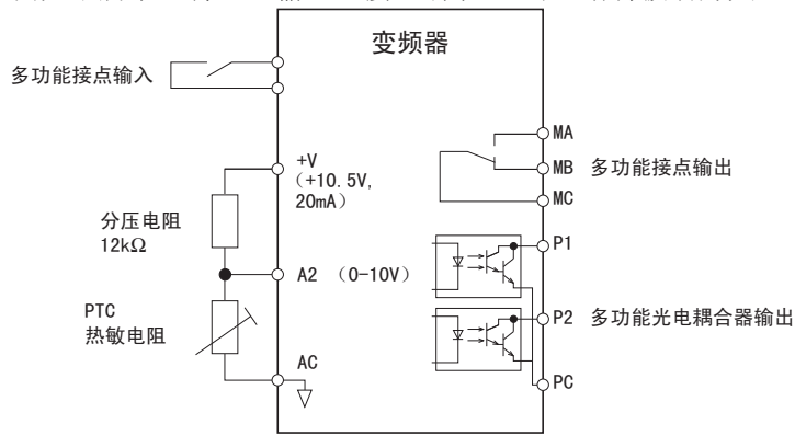
图 5.70 电机过热保护时的相互连接图 (PTC 输入的连接)
