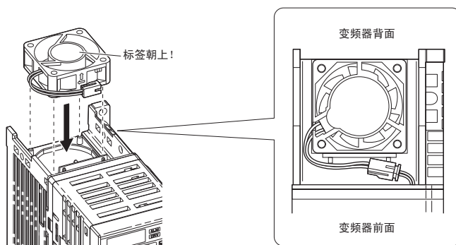
图 7.2 冷却风扇的安装方向
