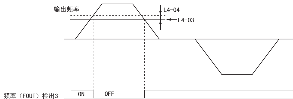
图 5.56 频率（FOUT）检出 3 的示例（L4-03 为正时）
