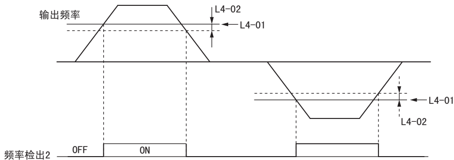
图 5.53 频率（FOUT）检出 2 的时序图
