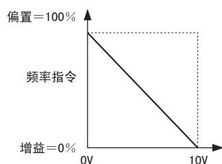
图 5.65 调整了逆变性场合的增益和偏置时的输出频率
