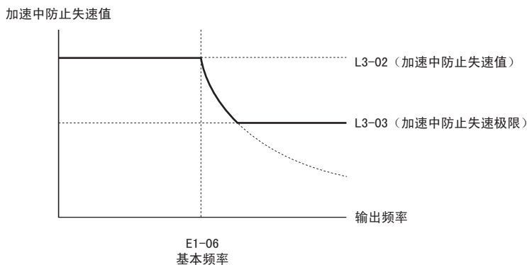
图 5.76 加速中防止失速值 / 极限
