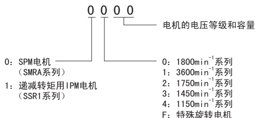
图 5.38 电机代码 (PM 用)
