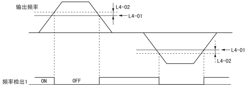
图 5.52 频率（FOUT）检出 1 的时序图
