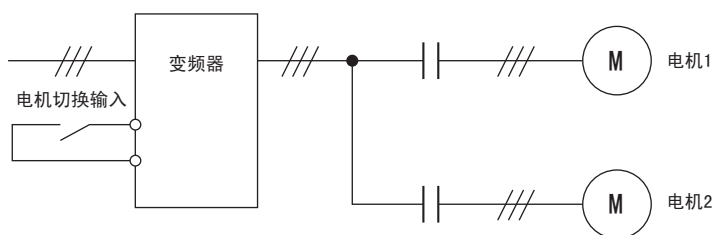
图 5.45 电机的切换
