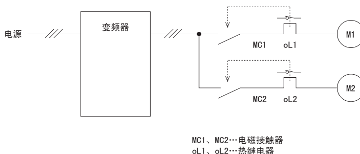
图 5.68 连接多台电机时的回路构成示例
