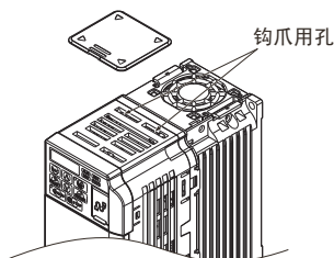
图 3.14 上部外罩的安装
