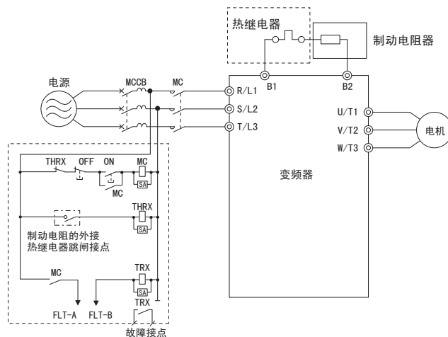
图 3.33 制动电阻器的连接
