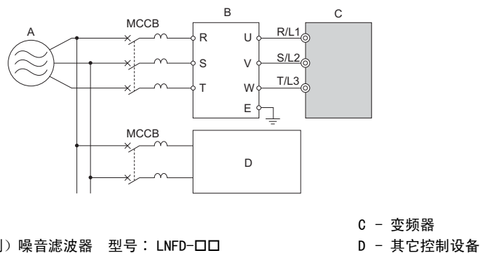
图 8.6 输入侧（一次侧）噪音滤波器的连接示例（三相 200V/400V）
